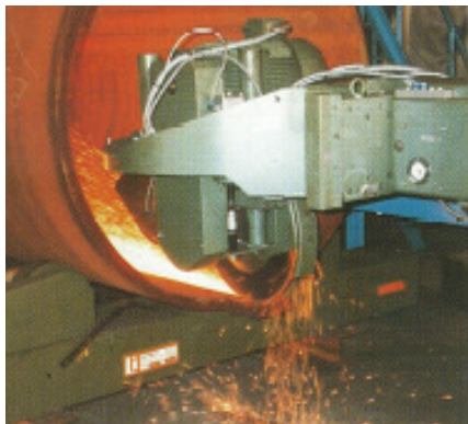
Schleifen der Wurzelseite an einer längs verlaufenden Schweissnaht innen und aussen.
