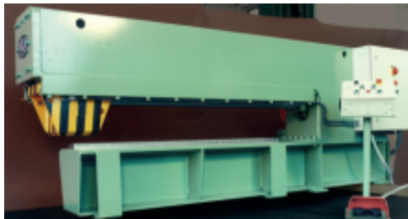
Längsnahtglättmaschine Typ LGO-2000 offen Longitudinal seams trowel open
